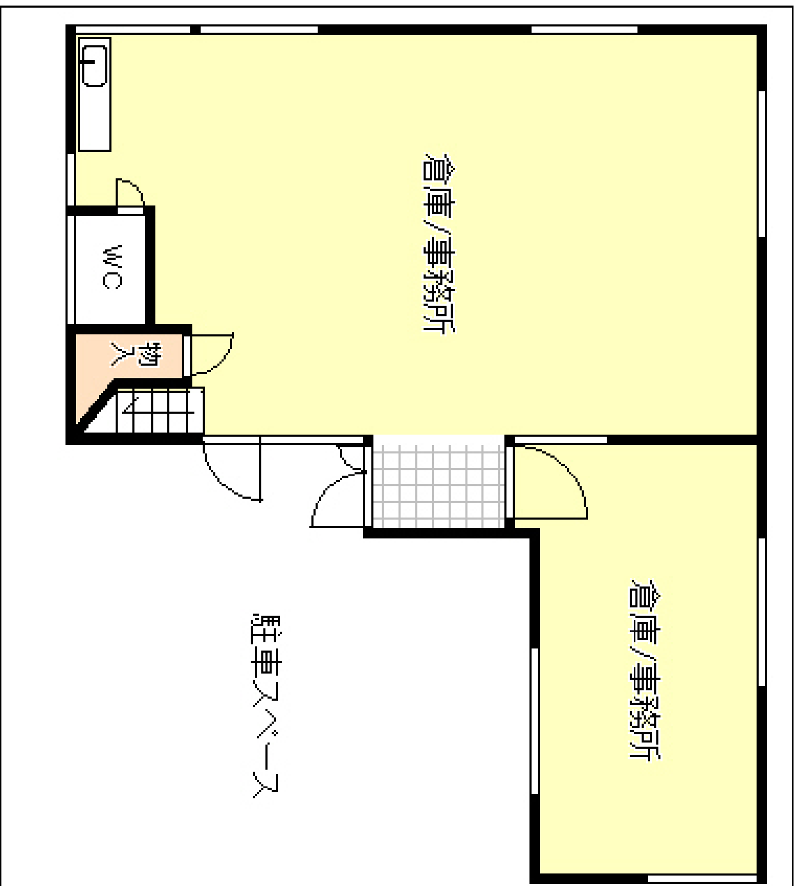
1階 平面図
